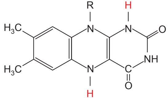
Reduzierte Form
