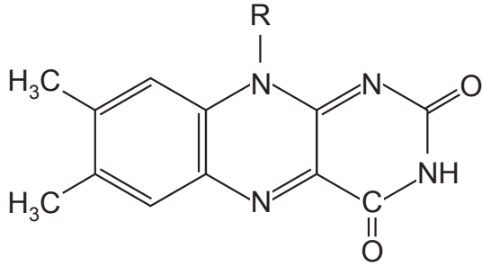
Oxidierte Form
