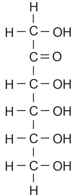
Ketose
