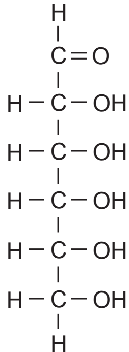
Aldose
