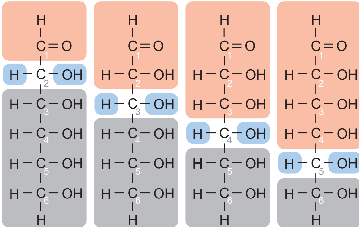
C2-Atom
