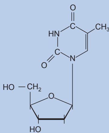
Desoxy-Thyminid (dT)
