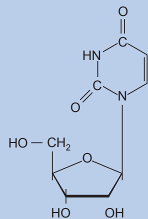
Uridin (U)
