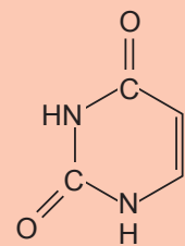
Uracil (Ura)
