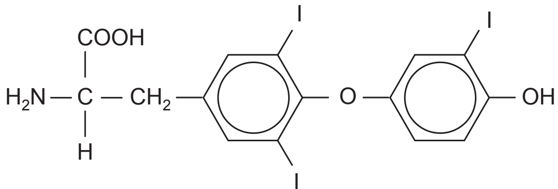
Trijodthyronin ( T_3 )
