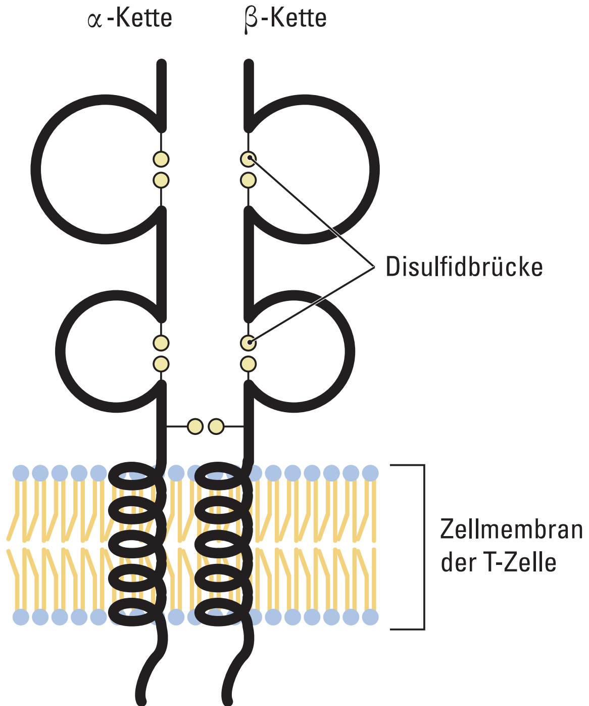
T-Zellrezeptor
