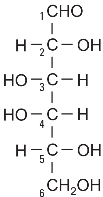
D-Galaktose
