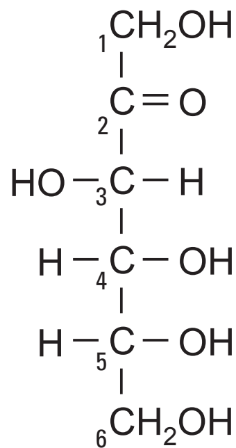
D-Fructose
