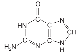
Guanin (Gua)
