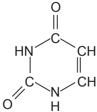
Uracil (Ura)
