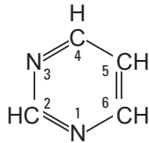
Pyrimidin Basen
