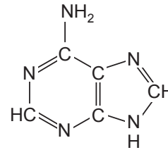
Adenin (Ade)
