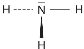
Ammoniak
