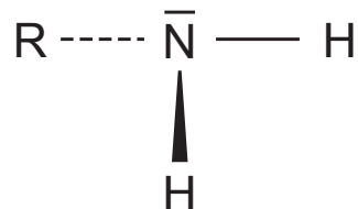
primäres Amin
