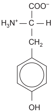
Tyrosin (Thr)
