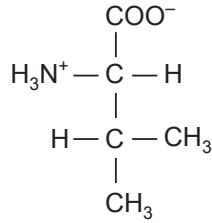
Valin (Val)*
