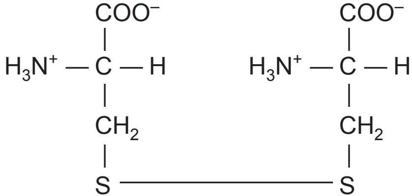
Disulfidbrücke
