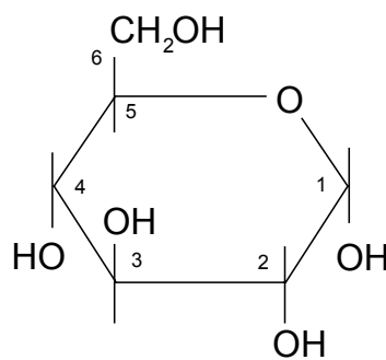
Haworth- Projektion
