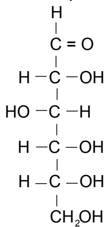
Fischer Projektion
