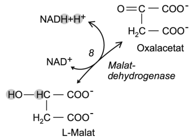
Abb. 43: Citratcyclus Schritt 8
