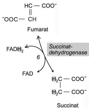
Abb. 41: Citratcyclus Schritt 6
