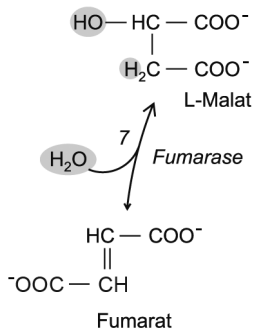
Abb. 42: Citratcyclus Schritt 7
