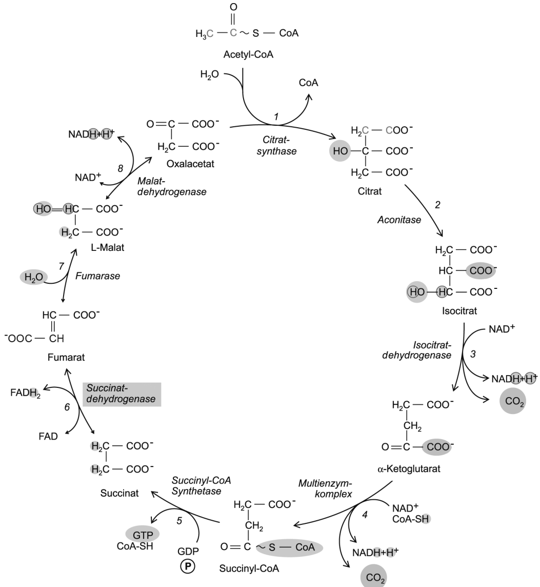
Abb. 45: Citratcyclus gesamt
