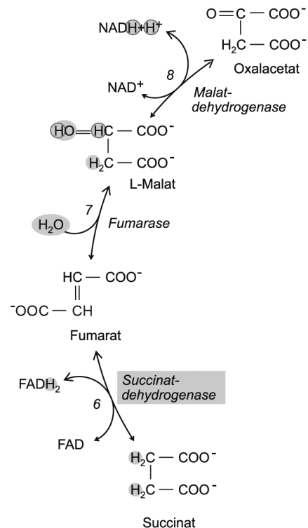
Abb. 44: Citratcyclus Teil 2
