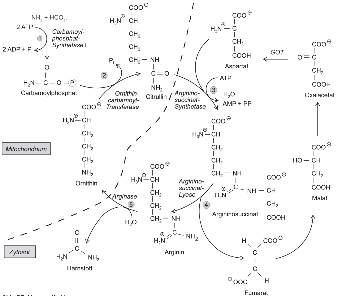
Abb. 37: Harnstoffzyklus
