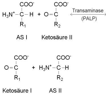
Abb. 28: Transaminierung
