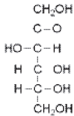
D-Fructose
