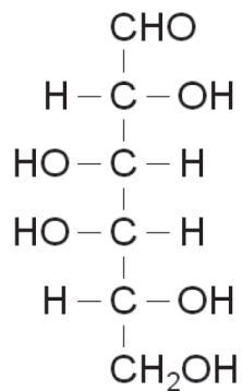
D-Galaktose
