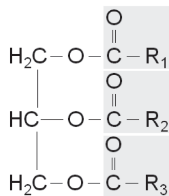
Triglycerid
