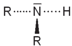
sekundäres Amin
