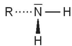
primäres Amin
