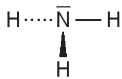
Ammoniak
