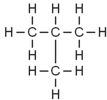
Isobutan
