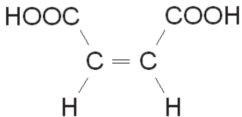
Maleinsäure (Cis-Isomer)
