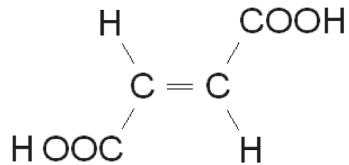
Fumarsäure (Trans-Isomer)
