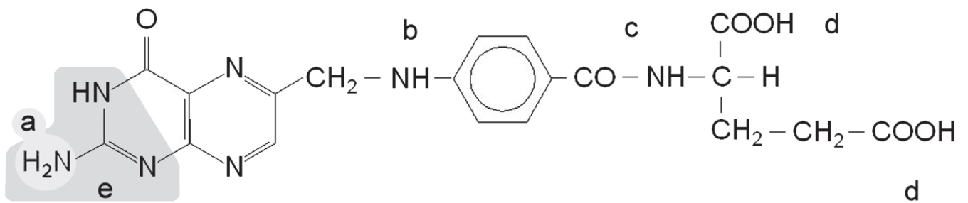
Folsäure
