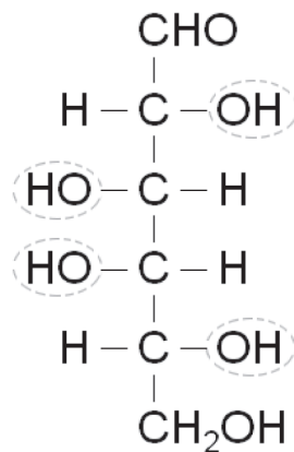
D - Galaktose
