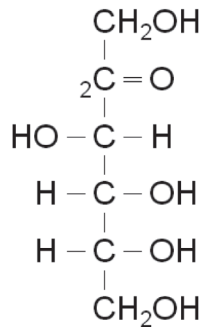
D-Fructose
