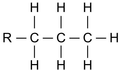
Alkylrest
