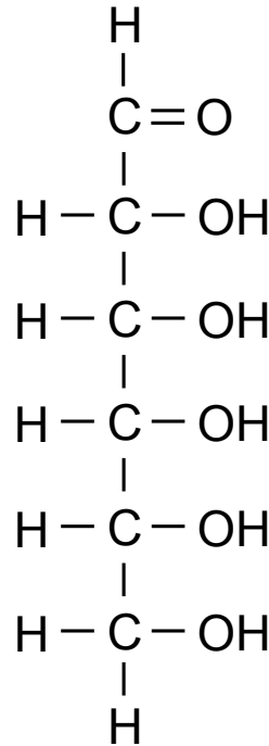
Aldose
