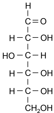
Fischer-Projektion
