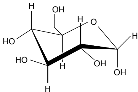
Sessel-Projektion
