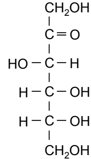
D-Fructose
