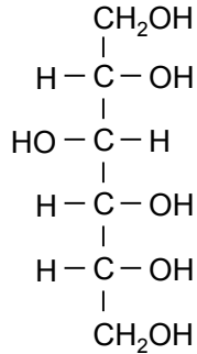
Sorbitol
