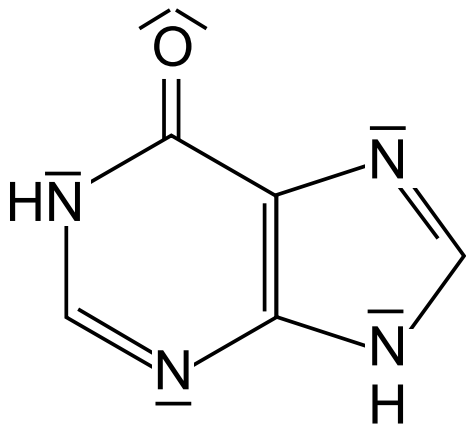
Ketoform
