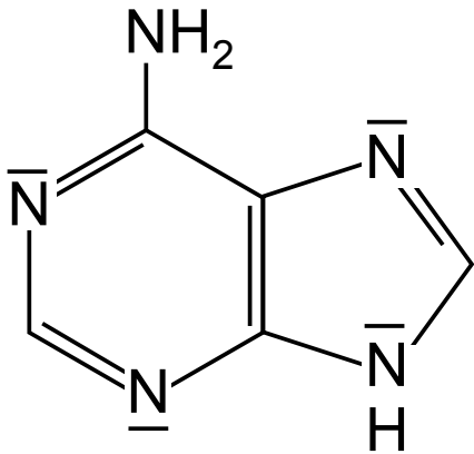
Aminoform
