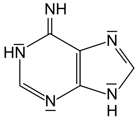
Iminoform
