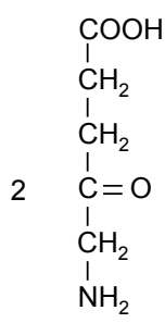
δ-Aminolävulinsäure
