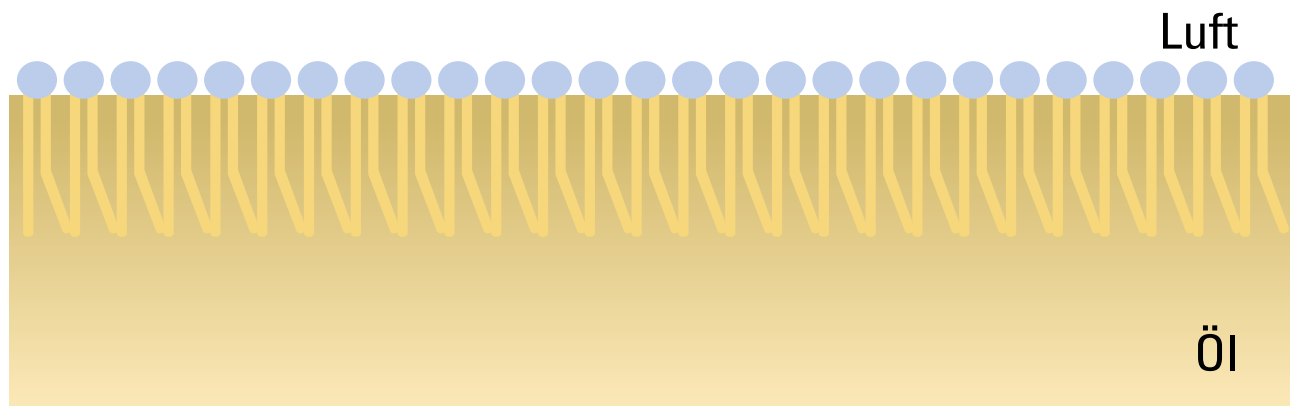
Oberflächenfilm (Monolayer)
