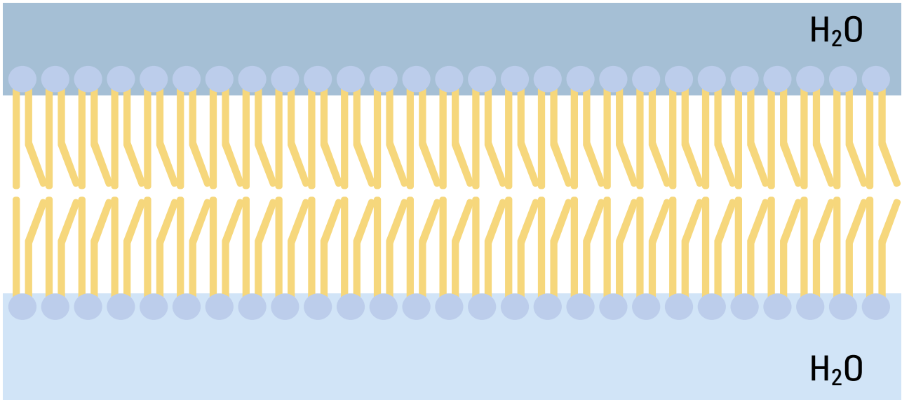
Doppelmembran (Bilayer)
