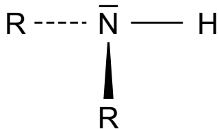
sekundäres Amin
