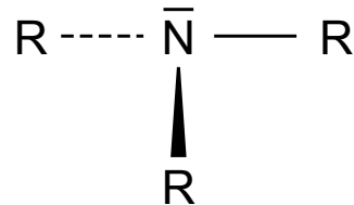
tertiäres Amin
