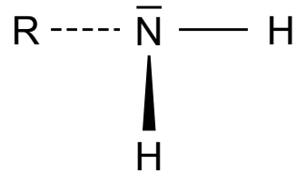
primäres Amin
