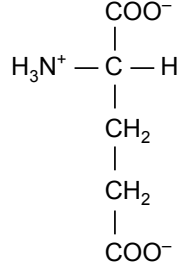
Glutaminsäure (Glu)
