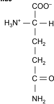
Glutamin (Gln)
