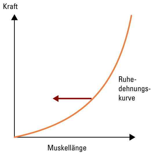
isotonische Kontraktion
