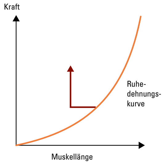
Anschlagszuckung
