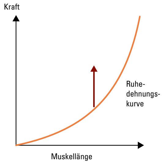
isometrische Kontraktion
