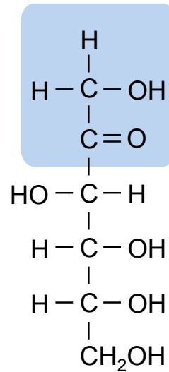
D-Fructose
