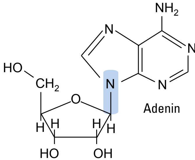
Ribose
