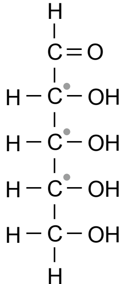
D-Ribose
