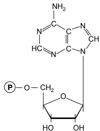
Adenosinmonophosphat AMP
