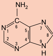
Adenin (Ade)
