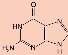
Guanin (Gua)
