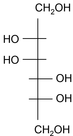
Mannitol
