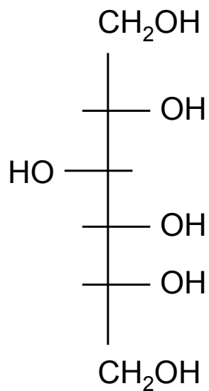
Sorbitol
