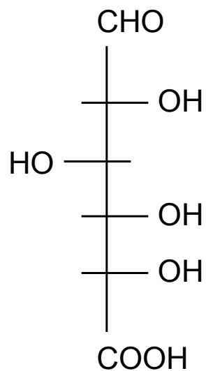
D-Glucuronsäure
