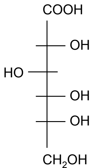
D-Gluconsäure
