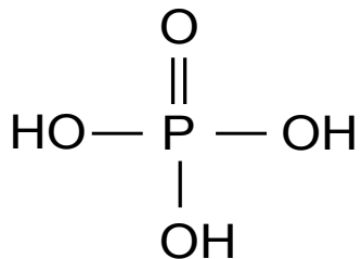
Phosphorsäure
