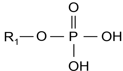
-monoester
