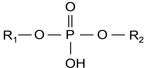
-diester
