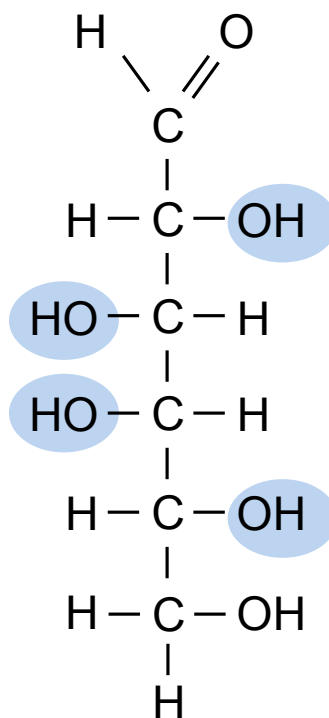
D-Galaktose
