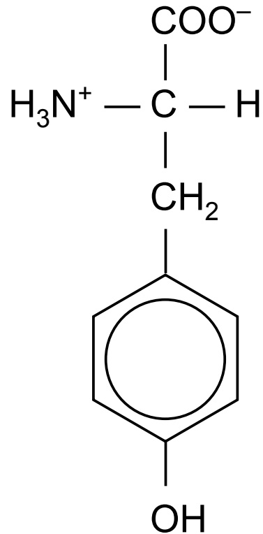
Tyrosin
