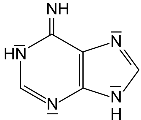
Iminoform
