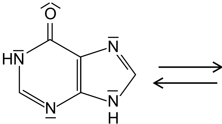
Ketoform
