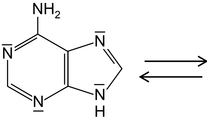
Aminoform
