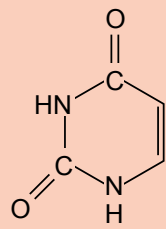
Uracil (Ura)
