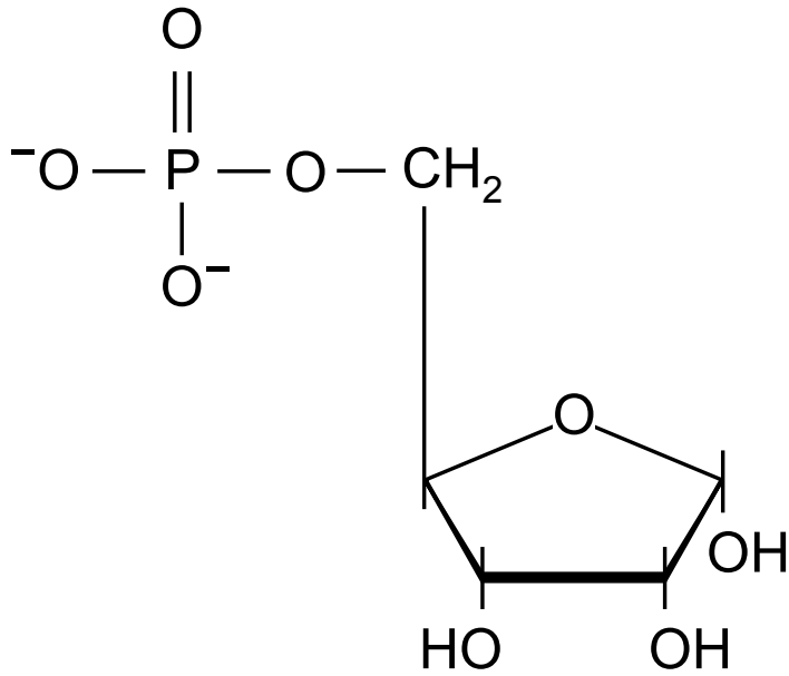
D-Ribose-5-Phosphat
