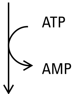
D-Ribose-5-Phosphat
