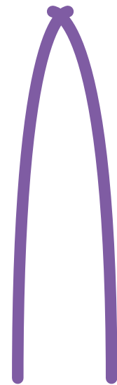
akro- zentrisch
