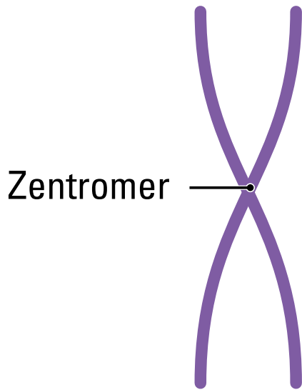
meta- zentrisch
