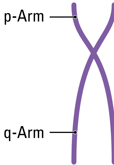
submeta- zentrisch
