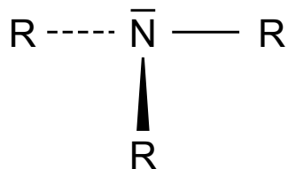
tertiäres Amin
