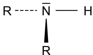
sekundäres Amin
