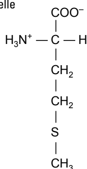
Methionin (Met)*
