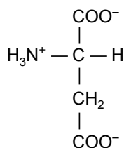
Asparaginsäure (Asp)
